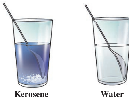
5.12 : Solubility
