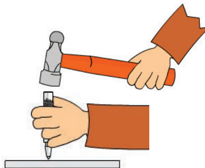
5.9 : Hardness
