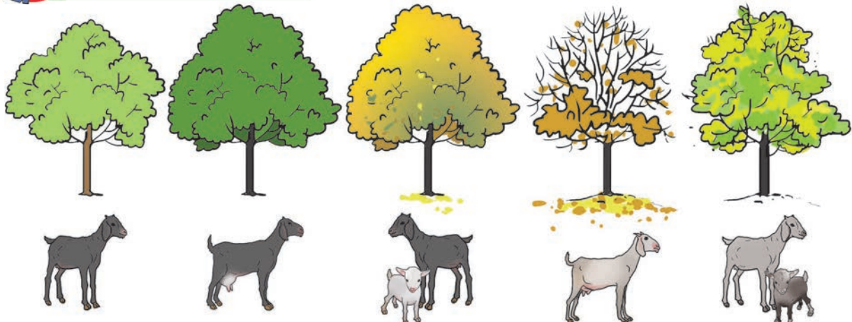
2.12 : Lifespan
