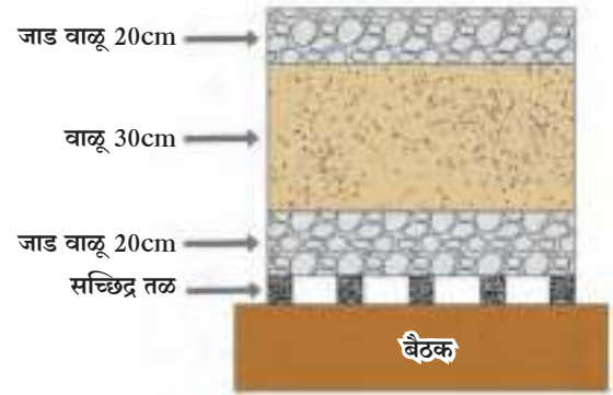
2.4.3 वाळूची गाळणी
