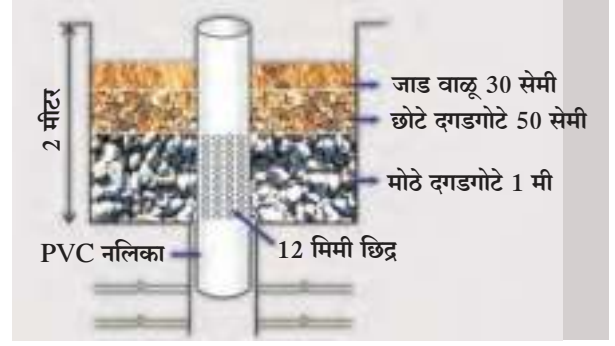
2.4.9 कूपनलिका रचना
