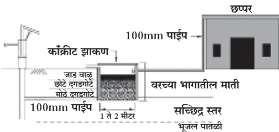
2.4.8 कूपनलिकेचे पुनर्भरण
