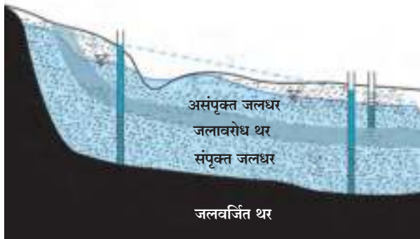
1.3.10 जलवर्जित थर
