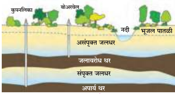
1.3.9 जलावरोध थर
