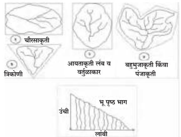
1.3.1 पाणलोट आकार
