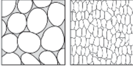
1.4.2 काळा पाषाण
