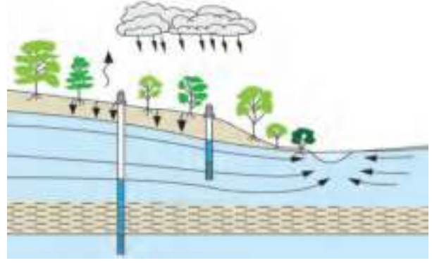
1.3.5 भूपृष्ठाखालील थर
